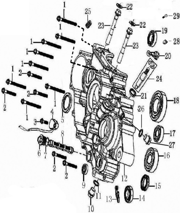
左曲轴箱 LEFT CRANKCASE
