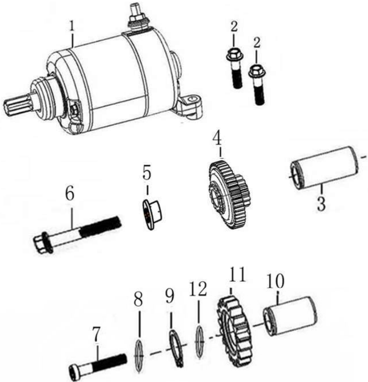
电启动机构
