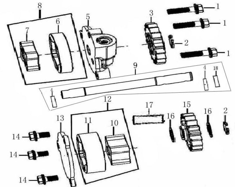
机油泵部件 OIL PUMP
