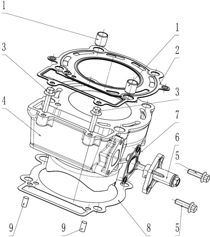
气缸体部件 CYLINDER ASSEMBLY
