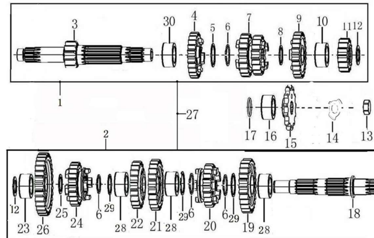
主副轴组合 TRANSMISSION MAIN, COUNTER SHAFT
