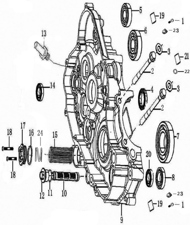
右曲轴箱 RIGHT CRANKCASE
